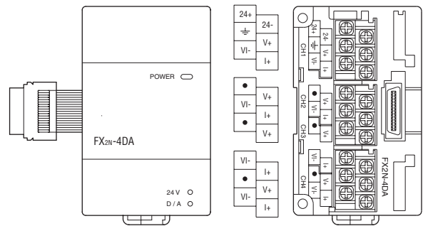
FX2N-4DA
