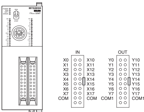
FX2NC-32MT-D/UL
