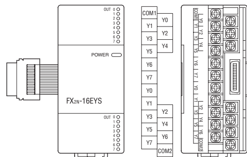
FX2N-16EYS-ES/UL
