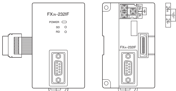
FX2N-232IF
